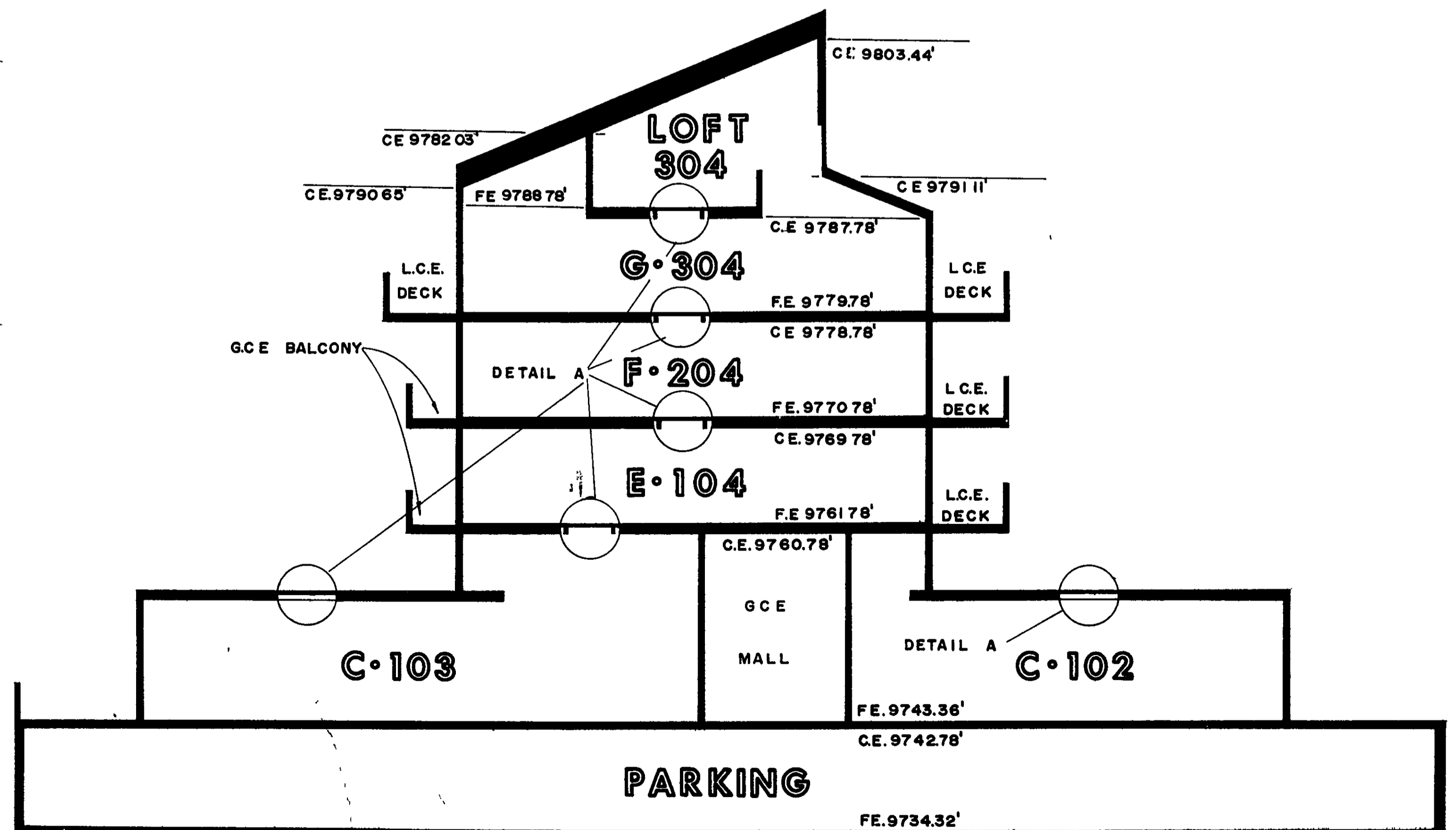
SECTION D-D
